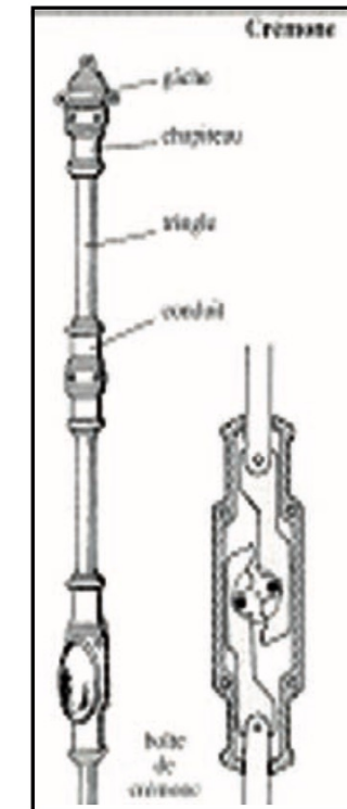
CREMONES
