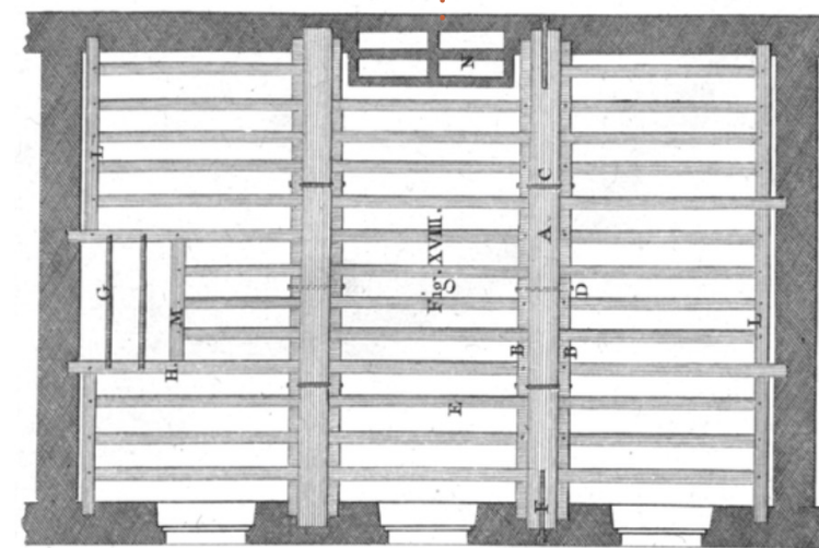
Plancher à la française plafonné sans retombée
