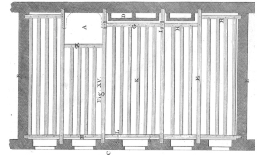
Plancher à système d'enchevêtreure :
