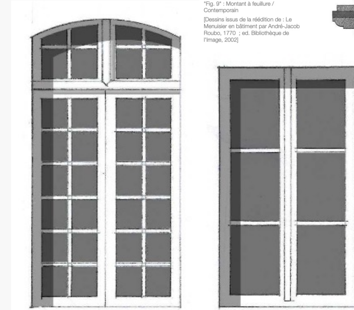
Le 18 e siècle - La fenêtre moderne
